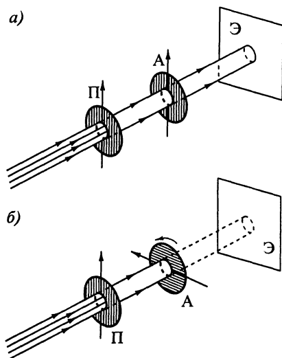
Рис. 1.4. Схема опыта для наблюдения поляризации света
