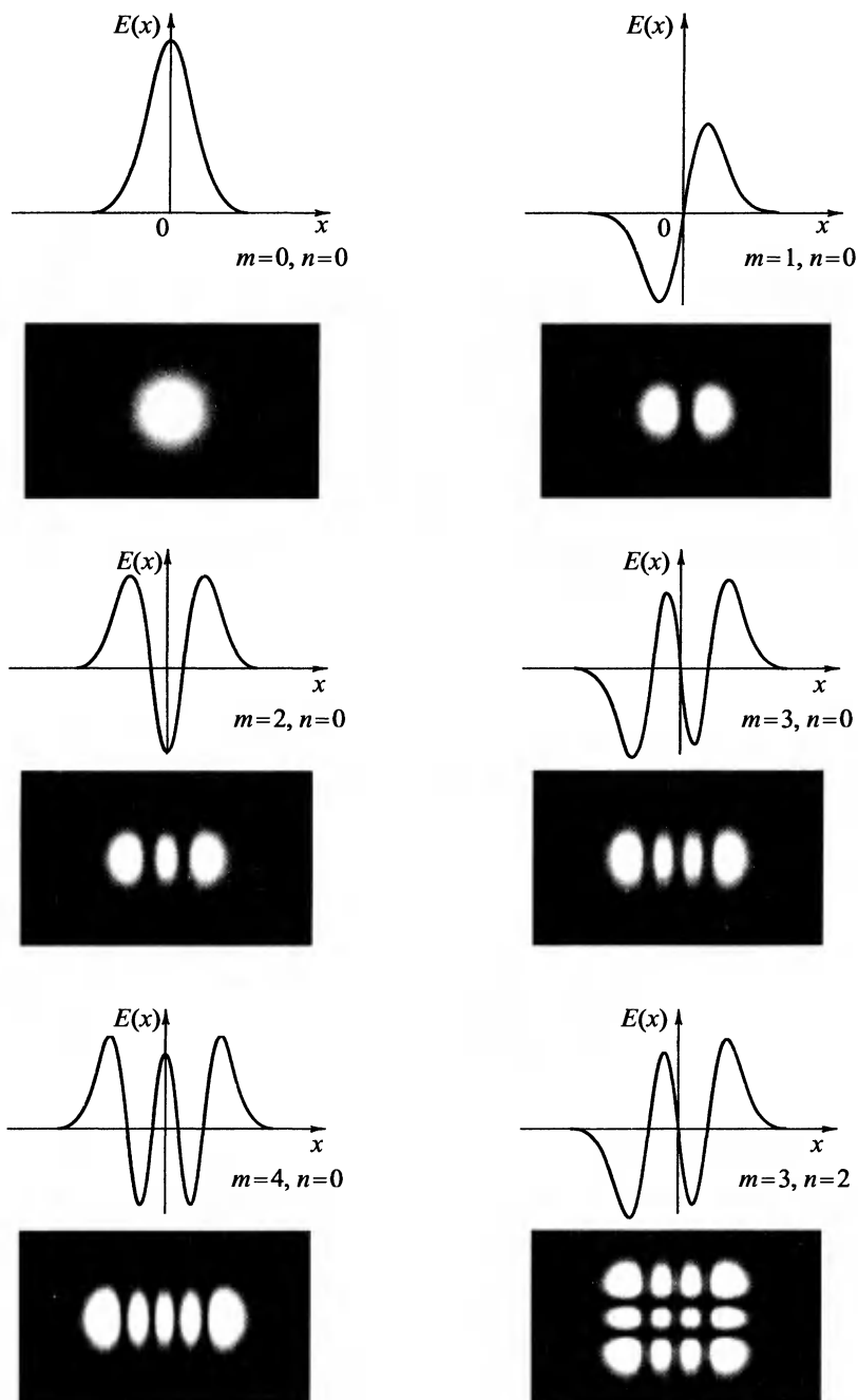
Рис. 9.5. Распределение амплитуды поля по поперечному сечению пучка и вид картины, наблюдаемой при освещении экрана лазерным пучком, для некоторых поперечных мод низкого порядка
