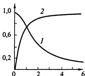
Рис. 6.41. Отношение разрешающей силы к ее значению при бесконечно узкой щели (1) и интенсивность в центре линии (2) в зависимости от ширины входной щели (по оси абсцисс отложено отношение ширины входной щели к ширине нормальной щели)
