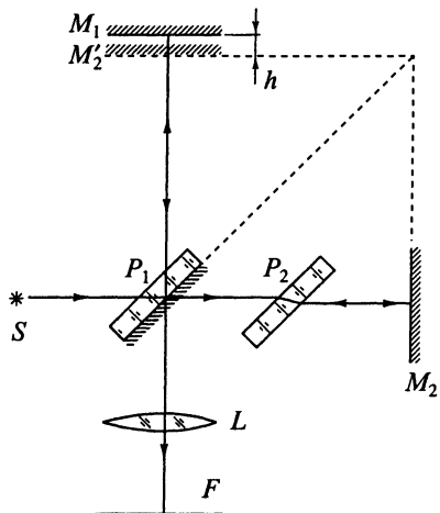
Рис. 5.11. Схема интерферометра Майкельсона
