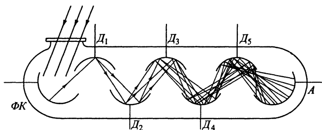
Рис. 9.12. Принципиальная схема фотоэлектронного умножителя (ФЭУ)
