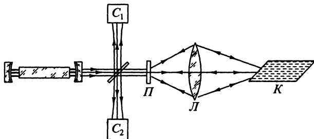
Рис. 10.6. Схема эксперимента по наблюдению обращения волнового фронта
