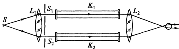
Рис. 5.26. Схема интерферометра Рэлея (вид сверху)
