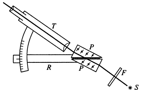
Рис. 3.9. Схема рефрактометра Аббе
