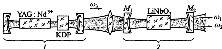
Рис. 10.4. Схема параметрического генератора света: 1 — лазер накачки с удвоителем частоты; 2 — нелинейный кристалл в оптическом резонаторе
