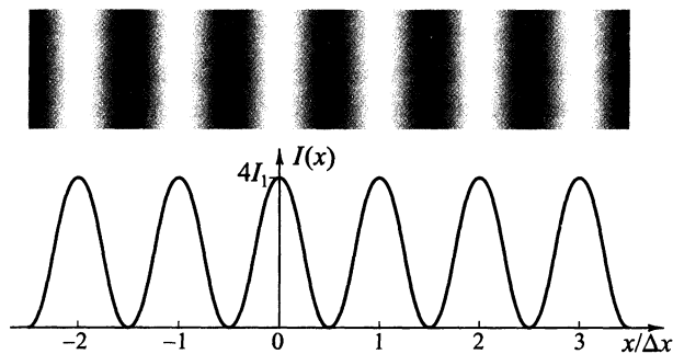
Рис. 5.3. Интерференционные полосы и график распределения интенсивности при интерференции двух монохроматических плоских волн одинаковой интенсивности
