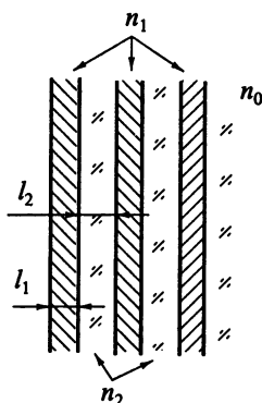
Рис. 5.33. Схема многослойного диэлектрического покрытия ( n_1 > n_0 , n_1 > n_2 , n_1 l_1 = n_2 l_2 = \lambda_0/4 )
