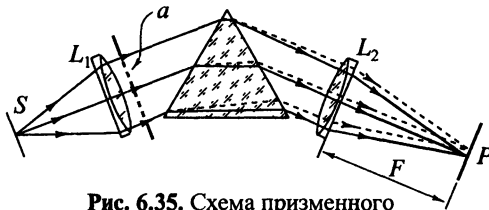
Рис. 6.35. Схема призматического спектрального прибора
