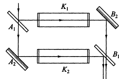
Рис. 5.28. Схема интерферометра Рождественского
