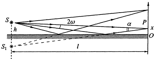
Рис. 5.24. Схема интерференционного опыта с зеркалом Ллойда
