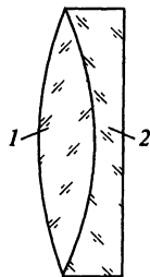
Рис. 7.27. Ахроматическая линза: 1 — крон; 2 — флинт
