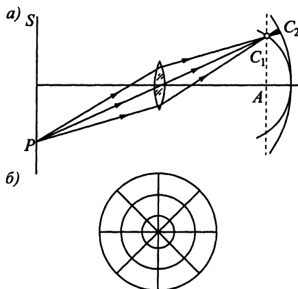
Рис. 7.25. Астигматизм наклонных пучков и кривизна поля изображения (а) и объект для испытания линз на астигматизм (б)
