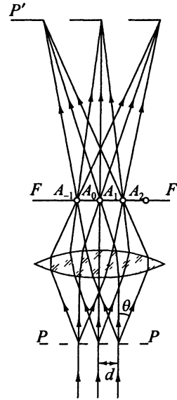
Рис. 7.34. К дифракционной теории образования изображения в микроскопе
