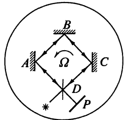
Рис. 8.9. Схема опыта Саньяка
