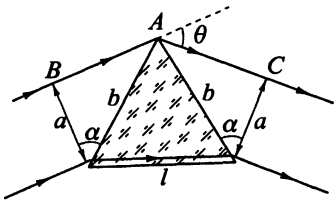
Рис. 6.40. К определению дисперсии и разрешающей способности призмы
