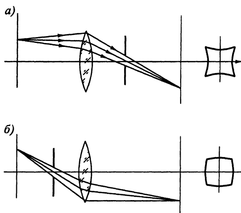
Рис. 7.26. Дисторсия изображения при разных положениях диафрагмы. Справа показаны изображения квадрата
