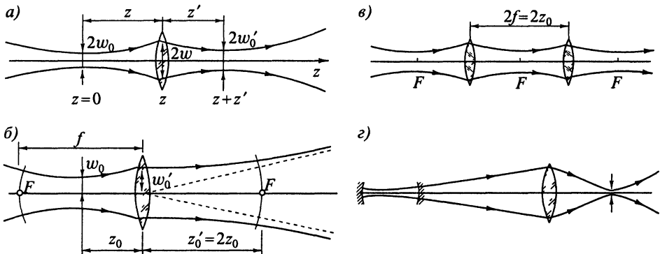
Рис. 6.30. Преобразование гауссова пучка при прохождении через линзу
