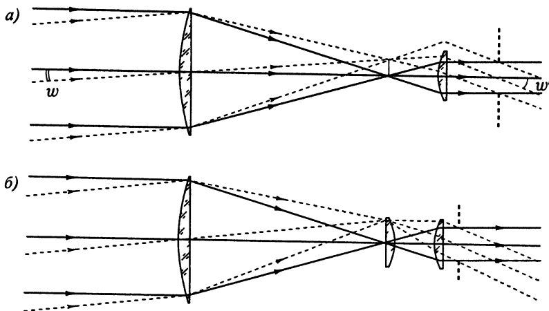
Рис. 7.19. Ограничение поля зрения оправой окуляра и связанное с этим затенение изображения (а) и применение полевой линзы для увеличения поля зрения (б)
