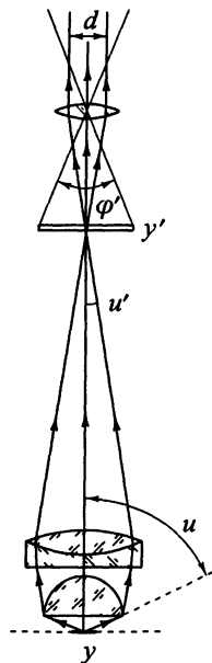
Рис. 7.29. К определению нормального увеличения микроскопа
