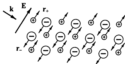
Рис. 2.5. Смещение положительных и отрицательных ионов кристалла в электрическом поле световой волны
