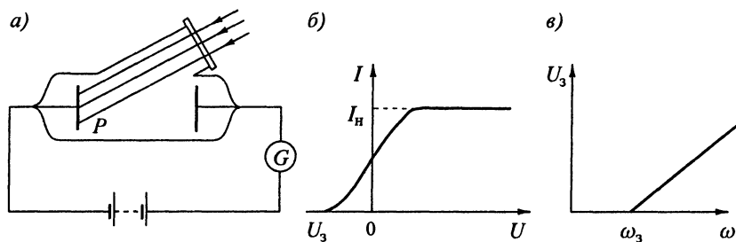
Рис. 9.10. Схема опыта для исследования фотоэффекта (а), вольт-амперная характеристика (б) и зависимость задерживающего напряжения от частоты (в)
