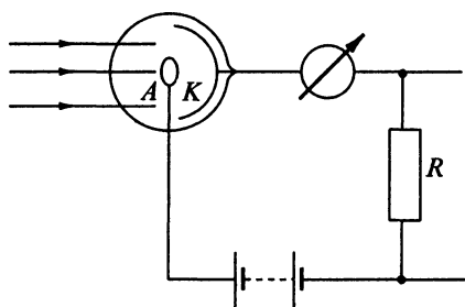
Рис. 9.11. Схема простейшего фотоэлемента
