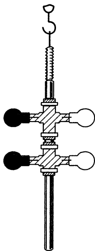
Рис. 3.18. Один из подвесов, использованных П. Н. Лебедевым в опытах по измерению светового давления
