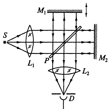
Рис. 5.30. К объяснению принципа действия Фурье-спектрометра
