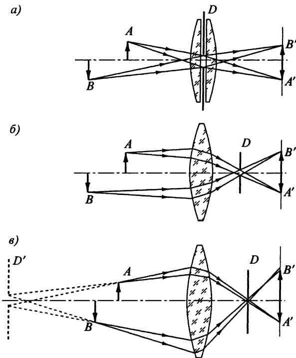
Рис. 7.18. Влияние положения апертурной диафрагмы D оптической системы на характер перспективы: нормальной (а); телецентрической (б); гиперцентрической (в) перспективы
