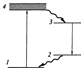
Рис. 9.7. Энергетическая диаграмма четырехуровневого лазера
