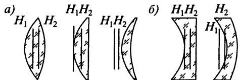
Рис. 7.11. Расположение главных плоскостей для толстых линз
