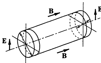
Рис. 8.13. Схема ячейки Фарадея
