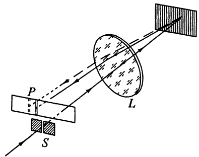
Рис. 6.36. Автоколлимационная схема спектрального прибора
