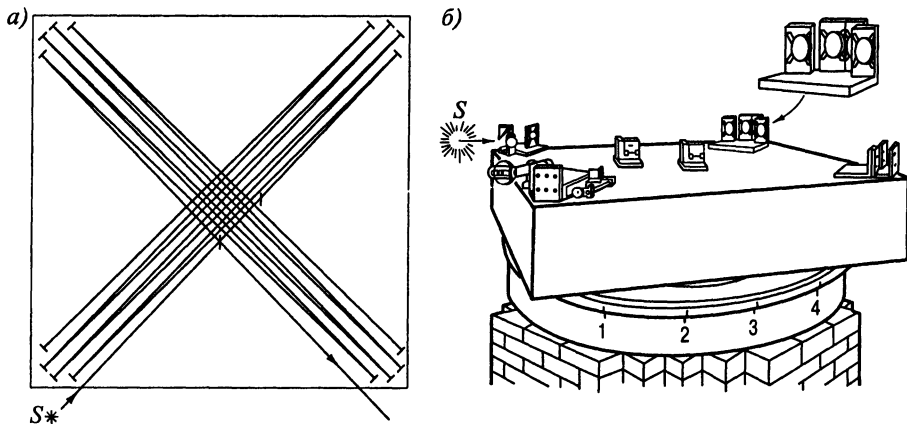
Рис. 8.4. Оптическая схема (а) и общий вид (б) интерферометра Майкельсона
