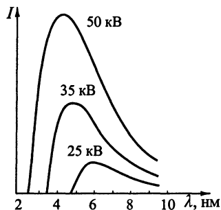
Рис. 9.14. Коротковолновая граница тормозного рентгеновского спектра
