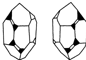
Рис. 2.10. Внешняя форма монокристаллов право- и левовращающего кварца. Вторая модификация является зеркальным изображением первой
