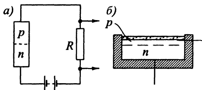
Рис. 9.13. Принципиальная схема (а) и устройство (б) фотодиода
