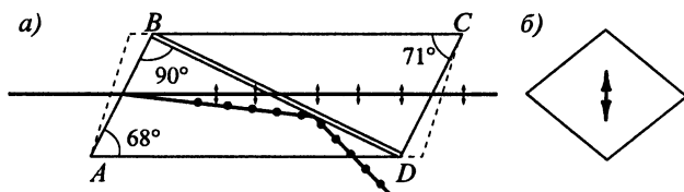
Рис. 4.13. Ход лучей в призме Николя (а) и вид призмы со стороны торцевой плоскости (б)
