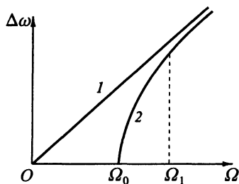
Рис. 8.12. Зависимость распределения частот встречных волн от угловой скорости \Omega : 1 — теоретическая линейная зависимость (8.23); 2 — экспериментальная кривая
