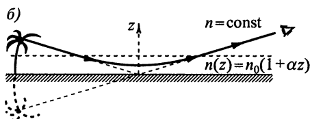
Рис. 7.1. Искривление лучей света в оптически неоднородной среде (а) и возникновение миража, обусловленное градиентом показателя преломления в нагретом слое воздуха, прилегающем к земле (б)
