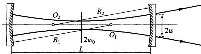
Рис. 6.28. Открытый оптический резонатор
