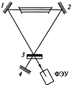
Рис. 8.11. Кольцевой лазер с трехзеркальным резонатором
