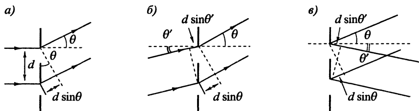
Рис. 6.33. К вычислению разности хода волн от соседних штрихов решетки
