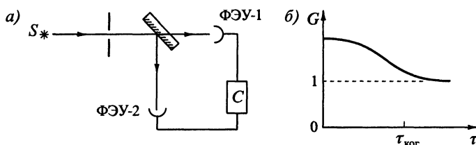
Рис. 5.19. Схема опыта Брауна и Твисса для измерения корреляционной функции интенсивностей G(\tau) и график G(\tau)
