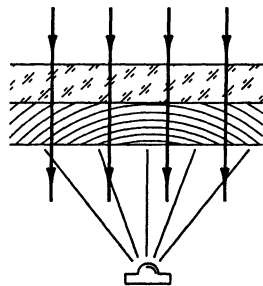
Рис. 7.40. Схема получения толстослойной голограммы по методу Ю. Н. Денисюка
