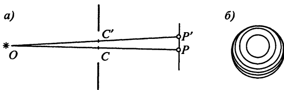
Рис. 6.8. Зоны Френеля для внеосевой точки наблюдения P'
