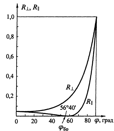
Рис. 3.7. Зависимость коэффициентов R_{\parallel} и R_{\perp} от угла падения на границе воздух–стекло
