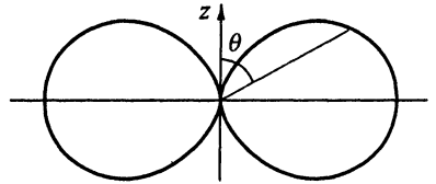
Рис. 1.17. Угловое распределение энергии, излучаемой осциллирующим диполем (диаграмма направленности)
