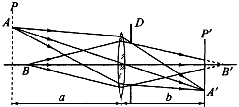
Рис. 7.16. К зависимости глубины резкости от ограничения световых пучков в оптической системе
