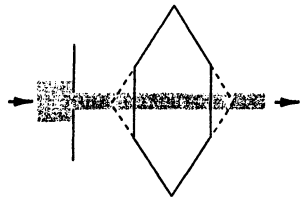
Рис. 4.3. Распространение света вдоль оптической оси кристалла исландского шпата
