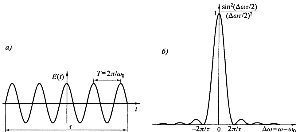
Рис. 1.21. Синусоидальный пучок волн конечной длительности \tau (а) и соответствующее распределение энергии по частотам (б)
