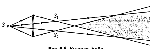
Рис. 5.8. Билинза Бийе
