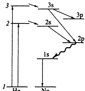
Рис. 9.9. Упрощенная схема энергетических уровней гелия и неона
