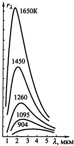
Рис. 9.1. Испускательная способность черного тела при разных температурах
