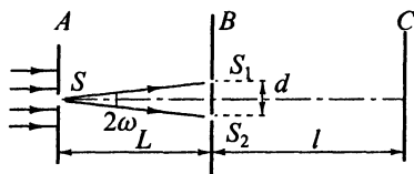
Рис. 5.5. Схема опыта Юнга
