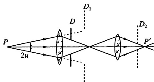
Рис. 7.17. Апертурная диафрагма ( D ), входной ( D_1 ) и выходной ( D_2 ) зрачки оптической системы
