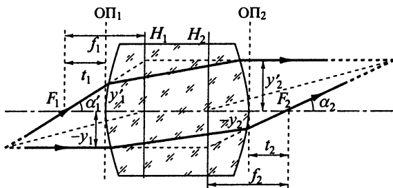
Рис. 7.10. К нахождению кардинальных точек оптической системы
