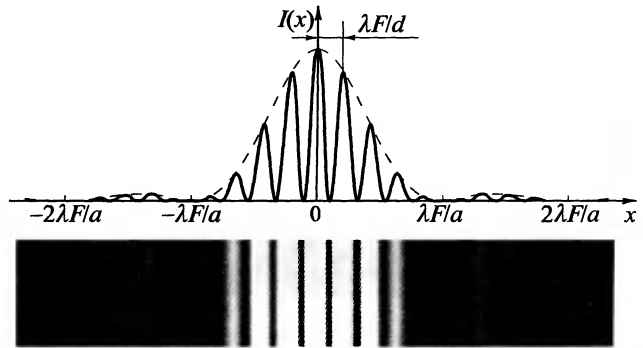
Рис. 6.25. Распределение интенсивности при дифракции Фраунгофера от двух одинаковых щелей. Центральная область сильно переэкспонирована для выделения слабых боковых полос
