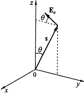
Рис. 4.8. К выбору направления осей координат
