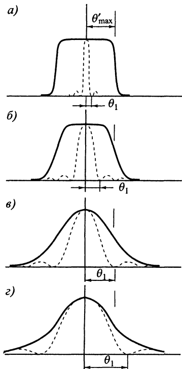
Рис. 6.20. Дифракция Фраунгофера на щели при протяженном источнике света
