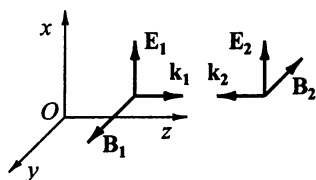
Рис. 1.9. Взаимная ориентация векторов \mathbf{E} , \mathbf{B} и \mathbf{k} в распространяющихся навстречу электромагнитных волнах линейной поляризации
