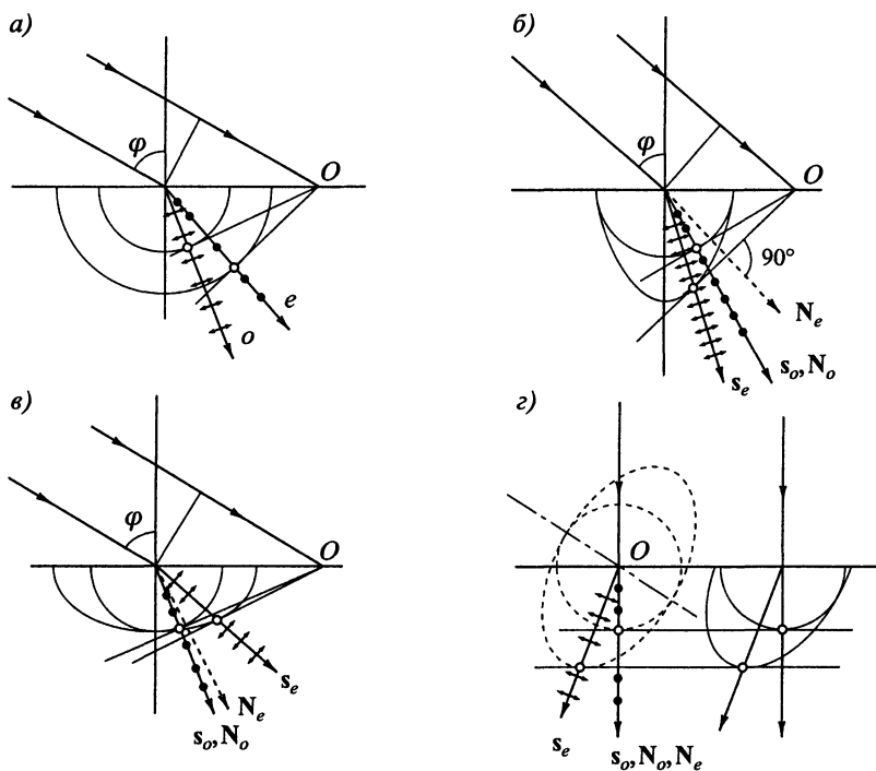
Рис. 4.12. Построение обыкновенного и необыкновенного лучей в одноосном кристалле при разных расположениях оптической оси (точками и стрелками показаны направления колебаний вектора \mathbf{E} )
