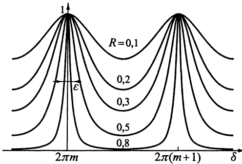
Рис. 5.32. Кривые распределения интенсивности в свете, проходящем через интерферометр Фабри–Перо
