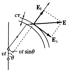
Рис. 1.15. Радиальная и поперечная составляющие вектора \mathbf{E} в области излома силовой линии
