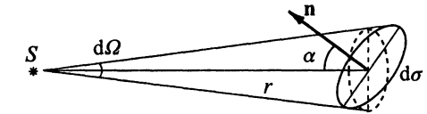
Рис. 1.27. К вычислению освещенности поверхности, создаваемой точечным источником
