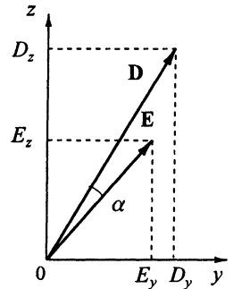
Рис. 4.7. Векторы \mathbf{D} и \mathbf{E} в анизотропной среде
