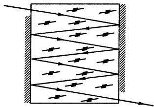
Рис. 2.7. Усиление эффекта поворота плоскости поляризации за счет удлинения пути при многократных отражениях
