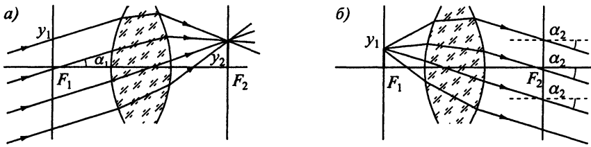
Рис. 7.12. Преобразование параксиальных лучей между фокальными плоскостями
