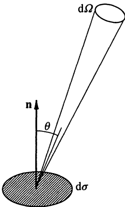
Рис. 1.28. К определению яркости излучающей поверхности
