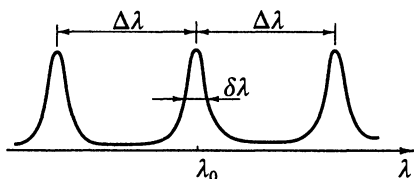
Рис. 5.35. Полосы пропускания интерференционного фильтра
