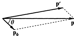
Рис. 9.17. Эффект Доплера при испускании фотона
