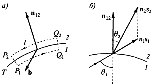
Рис. 7.2. К выводу закона преломления лучей света на искривленной границе раздела двух сред
