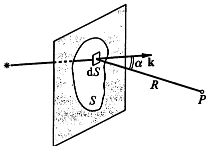
Рис. 6.1. К формулировке принципа Гюйгенса-Френеля
