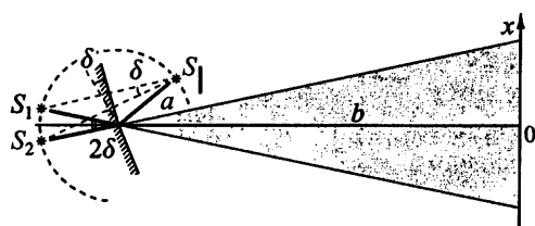
Рис. 5.6. Зеркала Френеля
