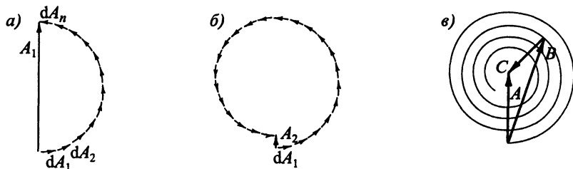
Рис. 6.4. Векторные диаграммы для результирующего колебания в точке наблюдения P : a — отверстие в экране открывает первую зону Френеля; b — две первые зоны; в — круглый экран перекрывает небольшое (нецелое) число зон Френеля
