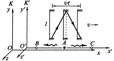
Рис. 8.5. Мысленные опыты, иллюстрирующие относительность одновременности событий и промежутков времени между событиями
