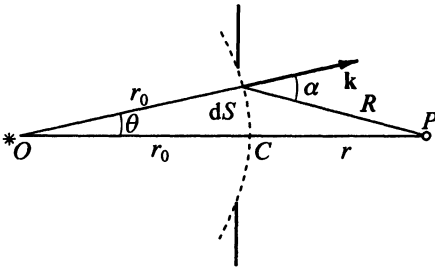
Рис. 6.2. К вычислению напряженности поля в точке наблюдения P
