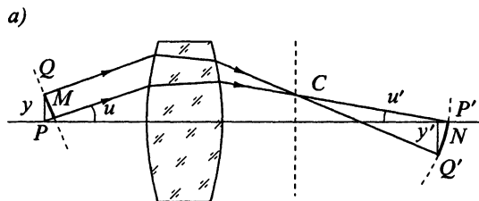
Рис. 7.24. К выводу условия синусов (а) и апланатические точки при преломлении на сферической поверхности (б)
