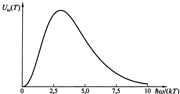
Рис. 9.2. График спектральной плотности равновесного теплового излучения (функции U_\omega(T) ), построенный по формуле Планка
