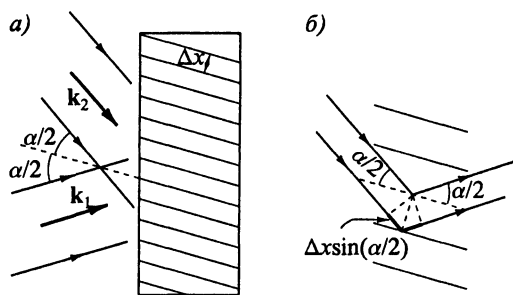
Рис. 7.39. К объяснению свойств толстослойных голограмм
