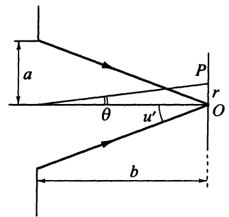
Рис. 7.30. К нахождению распределения интенсивности вблизи фокуса сходящегося пучка лучей
