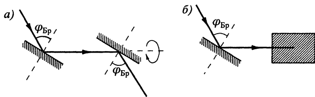
Рис. 3.6. Схема опыта, демонстрирующего поляризацию света, отраженного под углом Брюстера
