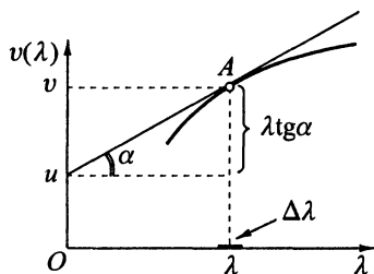
Рис. 2.17. Графическое определение групповой скорости из закона дисперсии
