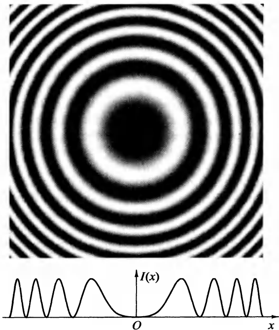
Рис. 5.14. Кольца Ньютона. Внизу показан график радиального распределения интенсивности
