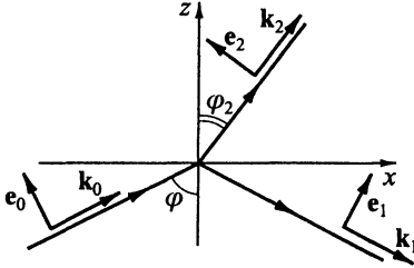
Рис. 3.3. Условный выбор положительных направлений векторов \mathbf{E} и \mathbf{B} для падающей, отраженной и преломленной волн
