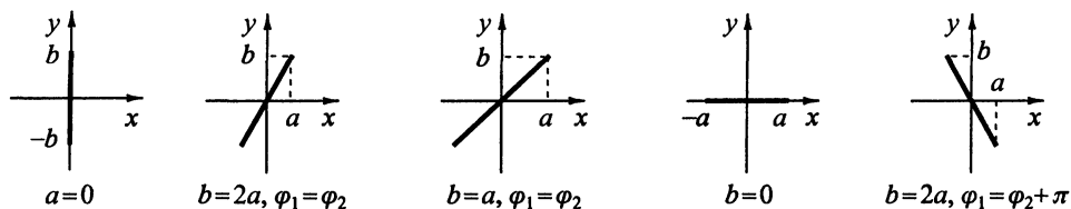
Рис. 1.5. Сложение двух поляризованных волн с ортогональными направлениями поляризации. При синфазных и противофазных складываемых колебаниях результирующая волна имеет линейную поляризацию
