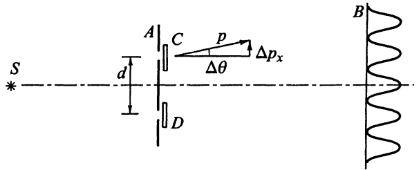
Рис. 9.18. Интерференционный опыт с двумя щелями
