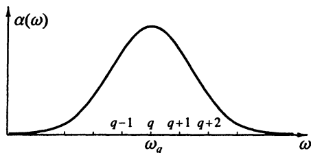
Рис. 9.4. Спектральный контур линии усиления
