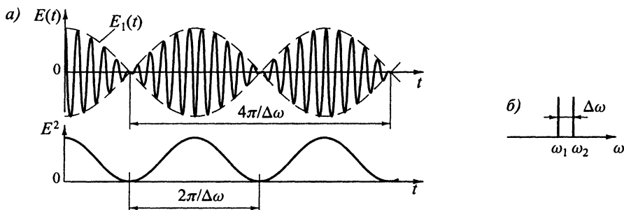
Рис. 1.20. Зависимость от времени напряженности поля и интенсивности при сложении двух монохроматических волн с близкими частотами и одинаковыми амплитудами
