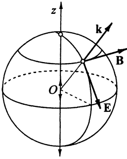
Рис. 1.16. Векторы \mathbf{E} , \mathbf{B} и \mathbf{k} в волновой зоне поля излучения осциллирующего заряда
