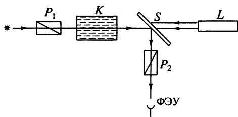
Рис. 4.16. Двойное лучепреломление в электрическом поле лазерного излучения
