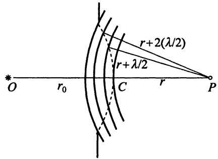
Рис. 6.3. Построение зон Френеля
