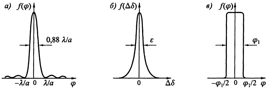
Рис. 6.37. Аппаратная функция спектрального прибора: а — спектрограф с призмой или дифракционной решеткой при узкой входной щели; б — интерферометр Фабри–Перо с узкой диафрагмой; в — аппаратная функция в случае широкой входной щели (или диафрагмы)
