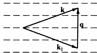
Рис. 10.5. Плоскости равных значений плотности в упругой волне с волновым вектором \mathbf{q}
