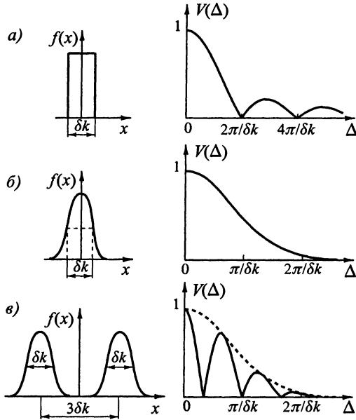
Рис. 5.17. Кривые видности, соответствующие различным спектральным распределениям интенсивности источника
