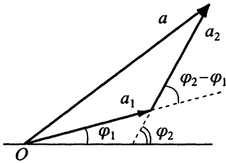
Рис. 5.1. Сложение гармонических колебаний с помощью векторной диаграммы
