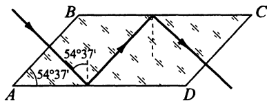
Рис. 3.13. Параллелепипед Френеля
