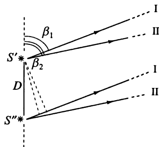
Рис. 5.20. К нахождению видности интерференционных полос в случае протяженного источника
