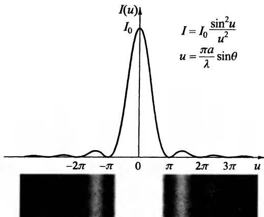
Рис. 6.18. Угловое распределение интенсивности при дифракции Фраунгофера на щели и фотография дифракционных полос. Центральный максимум на снимке сильно переэкспонирован для выявления слабых боковых максимумов
