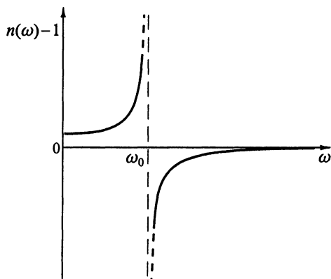
Рис. 2.1. Зависимость показателя преломления сильно разреженной среды от частоты (дисперсионная кривая) вдали от собственной частоты атомных осцилляторов \omega_0
