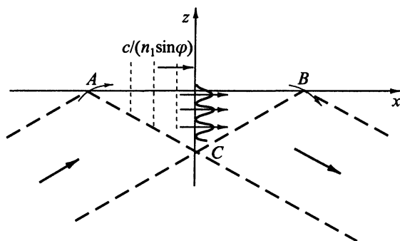
Рис. 3.12. Полное отражение пучка света с ограниченным поперечным сечением
