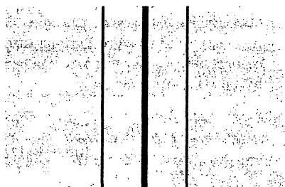
Рис. 1.26. Расщепление спектральной линии неона \lambda = 613,3 нм в магнитном поле 3,3 Тл при наблюдении поперек поля (фотографический негатив)
