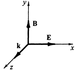
Рис. 1.1. Взаимное расположение векторов \mathbf{E} , \mathbf{B} и \mathbf{k} в бегущей электромагнитной волне
