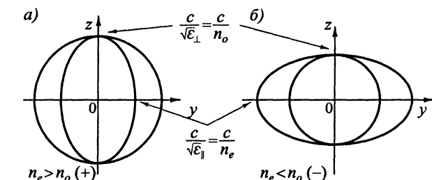
Рис. 4.9. Лучевые поверхности обыкновенной и необыкновенной волн в одноосных кристаллах
