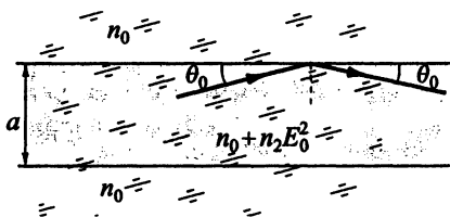
Рис. 10.1. К оценке порога самофокусировки
