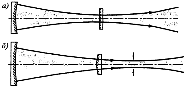
Рис. 6.29. Оптические резонаторы с плоским (а) и выпуклым (б) выходными зеркалами
