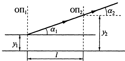
Рис. 7.7. К выводу матрицы преобразования параметров луча для оптического промежутка
