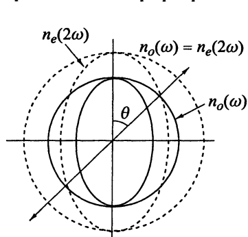
Рис. 10.3. Сечение поверхностей показателей преломления n_o и n_e в кристалле KDP и направление фазового синхронизма
