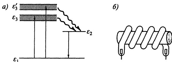
Рис. 9.6. Энергетические уровни иона хрома в рубине (а) и рубиновый стержень со спиральной лампой-вспышкой (б)
