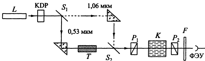
Рис. 4.17. Схема опыта для измерения времени релаксации искусственной анизотропии в электрическом поле
