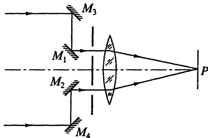
Рис. 5.25. Схема звездного интерферометра Майкельсона
