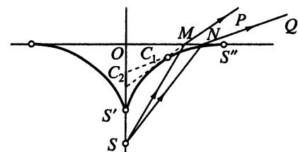
Рис. 7.21. Образование астигматических пучков при преломлении гомоцентрических пучков на границе раздела сред
