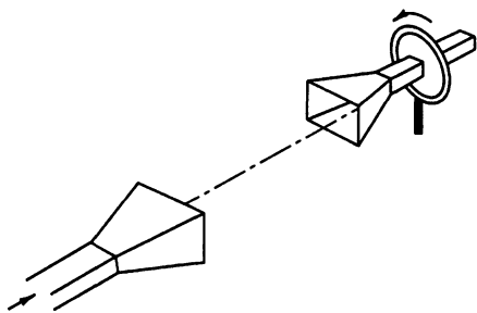
Рис. 1.3. Демонстрация поляризации электромагнитных волн в СВЧ-диапазоне
