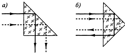
Рис. 3.11. Стеклянные призмы полного отражения
