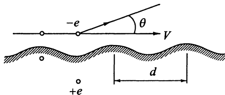
Рис. 2.20. Излучение, возникающее при движении заряда вдоль рельефной поверхности проводящей среды
