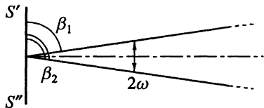
Рис. 5.22. Симметричное расположение протяженного источника
