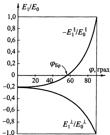
Рис. 3.4. Отношение амплитуд отраженной и падающей волн на границе воздух–стекло ( n = 1,5 )
