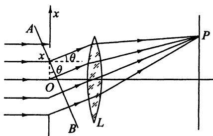
Рис. 6.17. Вторичная волна, приходящая в точку наблюдения P из точки волнового фронта с координатой x в отверстии экрана
