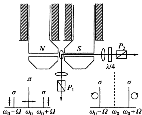
Рис. 1.25. Расщепление спектральной линии в эффекте Зеемана
