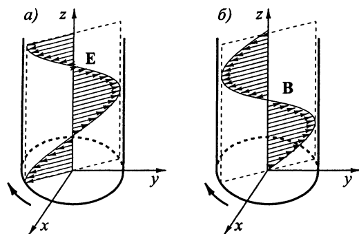
Рис. 1.12. Пространственное распределение электрического и магнитного полей в стоячей циркулярно поляризованной волне
