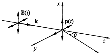
Рис. 2.14. К зависимости поляризации и интенсивности рассеянного света от угла рассеяния
