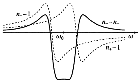
Рис. 2.9. Зависимость показателей преломления от частоты для волн с правой и левой круговыми поляризациями при распространении вдоль магнитного поля
