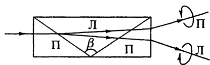
Рис. 2.11. Расщепление в призме Френеля пучка линейно поляризованного света на два пучка с правой и левой круговыми поляризациями
