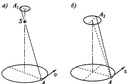
Рис. 8.1. Отклонение наблюдаемого положения звезды из-за параллакса (а) и аберрации (б)
