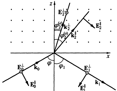
Рис. 4.10. Преломление и отражение плоской волны на границе одноосной среды
