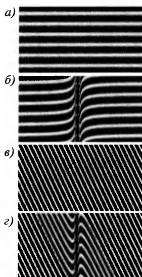
Рис. 5.29. Интерференционные полосы, развернутые в спектр, и крюки Рождественского
