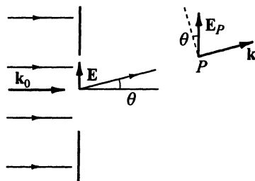
Рис. 6.15. Векторы напряженности электрического поля \mathbf{E} падающей волны в плоскости отверстия и дифрагировавшей волны \mathbf{E}_P в точке наблюдения P в приближении Френеля
