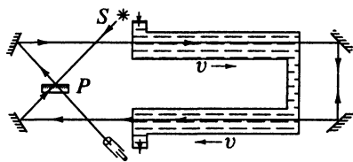
Рис. 8.2. Схема опыта Физо
