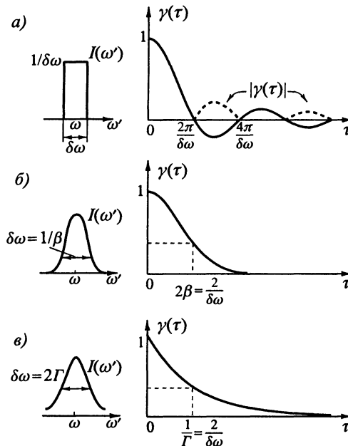
Рис. 5.18. Степень временной когерентности |\gamma(\tau)| , соответствующая различным спектральным распределениям интенсивности излучения
