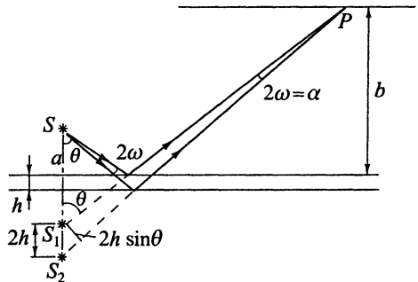
Рис. 5.9. Интерференция при отражении света двумя поверхностями тонкой пластинки
