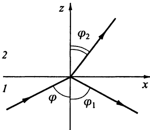
Рис. 3.2. Направления падающей, отраженной и преломленной волн на плоской границе раздела двух сред
