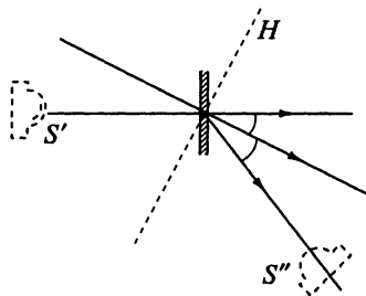
Рис. 7.38. Расположение изображений объекта при восстановлении голограммы
