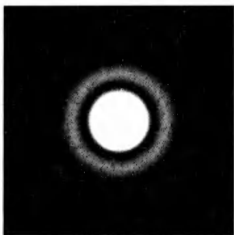
Рис. 6.23. Дифракция Фраунгофера от круглого отверстия. Центральная область сильно переэкспонирована для выявления слабых побочных максимумов
