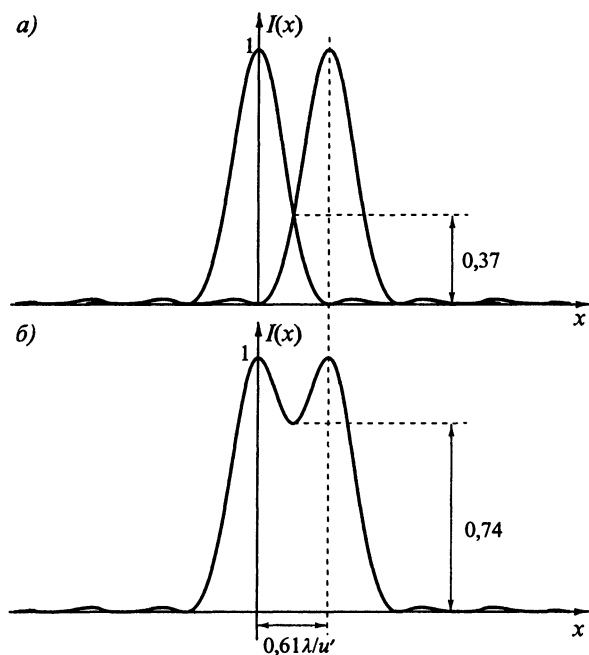
Рис. 7.31. Условный критерий разрешения изображений точечных некогерентных источников (критерий Рэлея)
