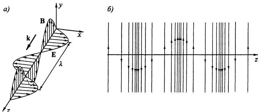
Рис. 1.2. Векторы \mathbf{E} и \mathbf{B} в монохроматической плоской волне в разных точках оси z в один момент времени ( а ) и соответствующая картина силовых линий электрического поля ( б ). Густота линий пропорциональна напряженности поля
