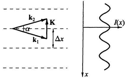
Рис. 5.2. Плоскости равных интенсивностей и освещенность экрана при интерференции плоских монохроматических волн
