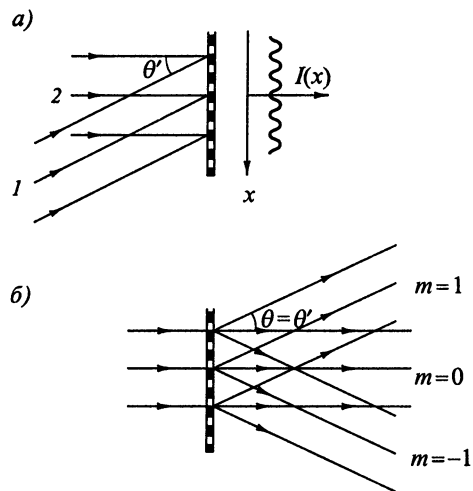
Рис. 7.35. Получение ( а ) и восстановление ( б ) голограммы плоской волны
