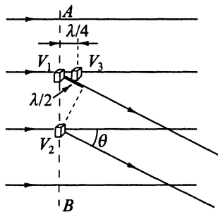
Рис. 2.12. К объяснению отсутствия рассеянного света в идеально однородной среде
