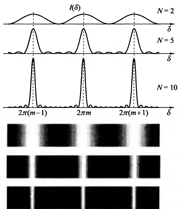
Рис. 6.32. Распределение интенсивности при двухлучевой и многолучевой интерференции одинаковых пучков (график функции \sin^2(N\delta/2)/\sin^2(\delta/2) при N , равном 2, 5 и 10)
