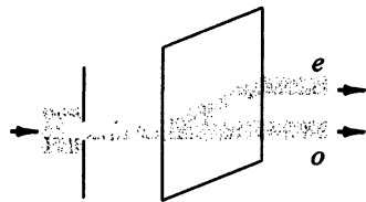
Рис. 4.2. Двойное лучепреломление света при нормальном падении неполяризованного света на естественную грань кристалла исландского шпата
