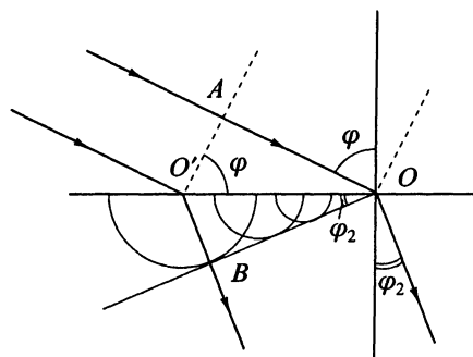
Рис. 4.11. Построение преломленной волны по принципу Гюйгенса (для изотропной среды)
