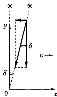
Рис. 8.7. К выводу формулы для аберрации света ( \sin \delta = v/c )
