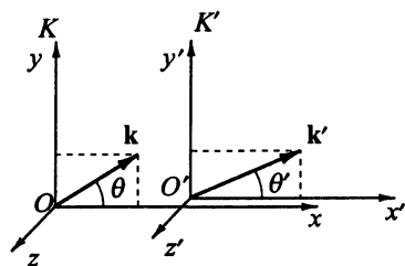
Рис. 8.8. Преобразование волнового вектора световой волны при переходе из одной системы отсчета в другую
