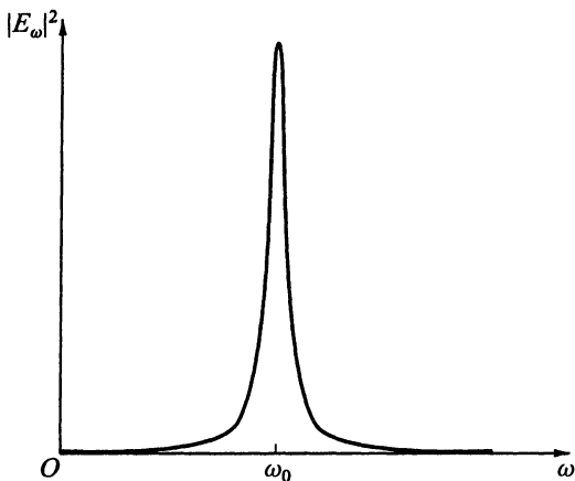
Рис. 1.23. Лоренцевский контур спектральной линии
