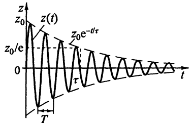
Рис. 1.18. Радиационное затухание колебаний излучающего электрона
