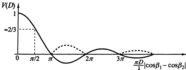
Рис. 5.21. Зависимость видности интерференционных полос от ширины D протяженного источника
