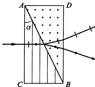
Рис. 4.14. Ход лучей в призме Волластона
