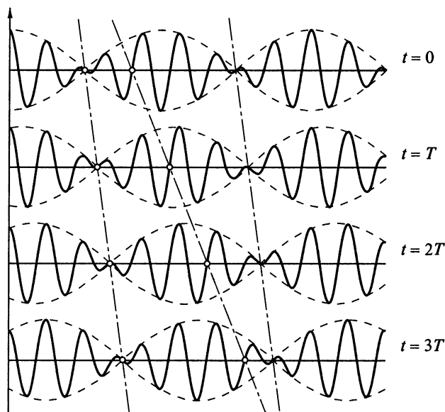
Рис. 2.15. Группы волн, возникающие при сложении двух волн с длинами \lambda и \lambda + \Delta\lambda
