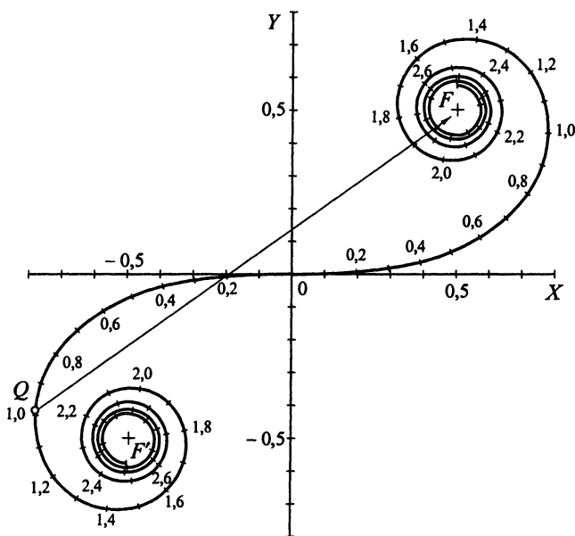
Рис. 6.11. Спираль Корню
