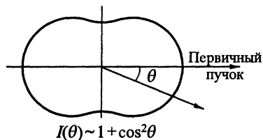
Рис. 2.13. Индикатриса рассеяния неполяризованного света в мутной среде
