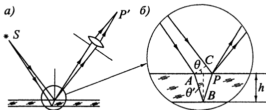
Рис. 5.12. Наблюдение полос, локализованных на поверхности тонкой пленки
