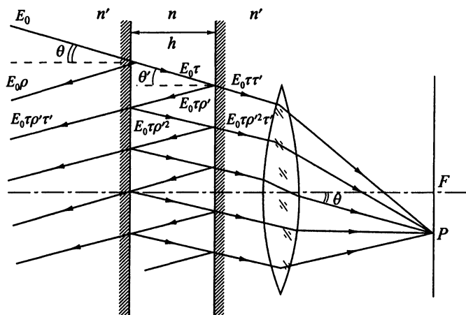
Рис. 5.31. Полосы равного наклона при многолучевой интерференции
