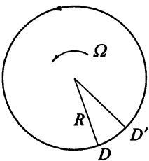
Рис. 8.10. К расчету запаздывания встречных волн
