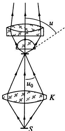
Рис. 7.33. К вопросу о когерентности освещения предмета в микроскопе
