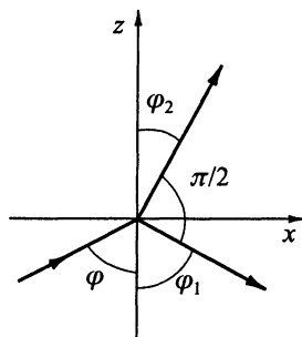
Рис. 3.5. К определению угла полной поляризации (угла Брюстера)
