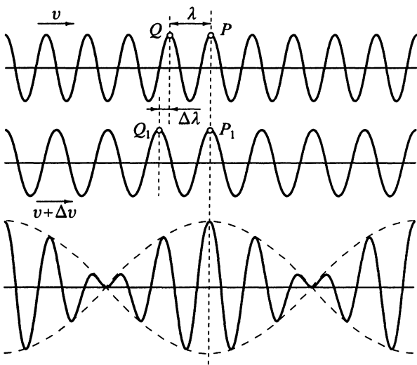
Рис. 2.16. К выводу формулы для групповой скорости волн
