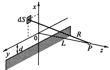
Рис. 6.9. К расчету дифракционной картины Френеля вблизи границы тени от прямолинейного края полубесконечного непрозрачного экрана
