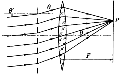
Рис. 6.31. Дифракция Фраунгофера на системе одинаковых параллельных щелей
