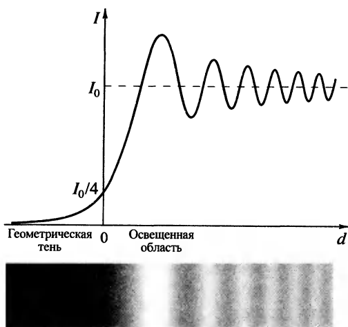
Рис. 6.12. Распределение интенсивности вблизи края геометрической тени прямолинейного полубесконечного экрана
