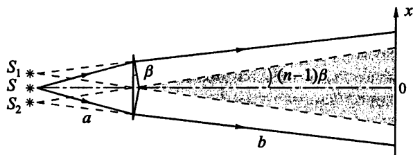
Рис. 5.7. Бипризма Френеля
