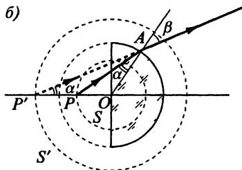
Рис. 7.24. К выводу условия синусов (а) и апланатические точки при преломлении на сферической поверхности (б)
