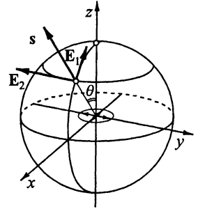
Рис. 1.19. К расчету поля излучения заряда, движущегося по окружности
