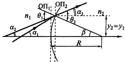
Рис. 7.8. К выводу матрицы преобразования параметров луча при преломлении на сферической поверхности
