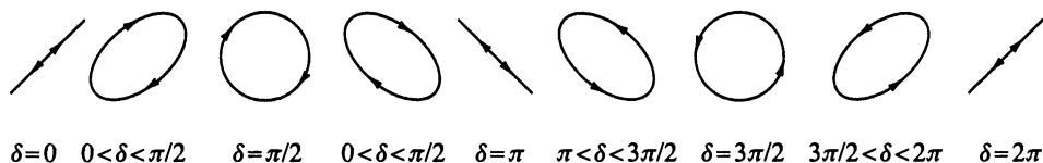
Рис. 1.7. Сложение взаимно перпендикулярных колебаний одинаковой амплитуды при разных фазах
