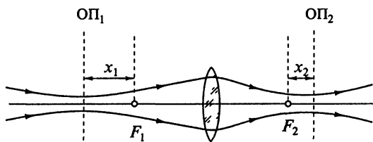
Рис. 7.15. Преобразование гауссова пучка при прохождении через линзу
