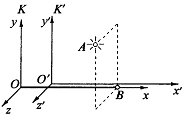
Рис. 8.6. К выводу преобразований Лоренца
