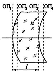
Рис. 7.9. Толстая линза
