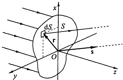
Рис. 6.21. К расчету дифракции Фраунгофера от отверстия
