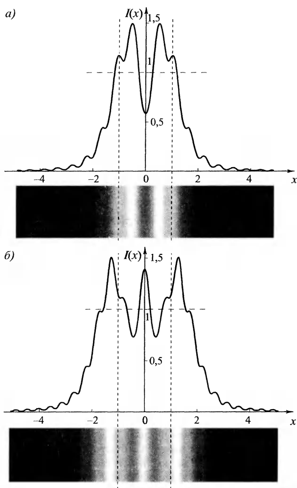
Рис. 6.13. Картины дифракции Френеля от щелей разной ширины. Штриховыми линиями показаны границы геометрической тени
