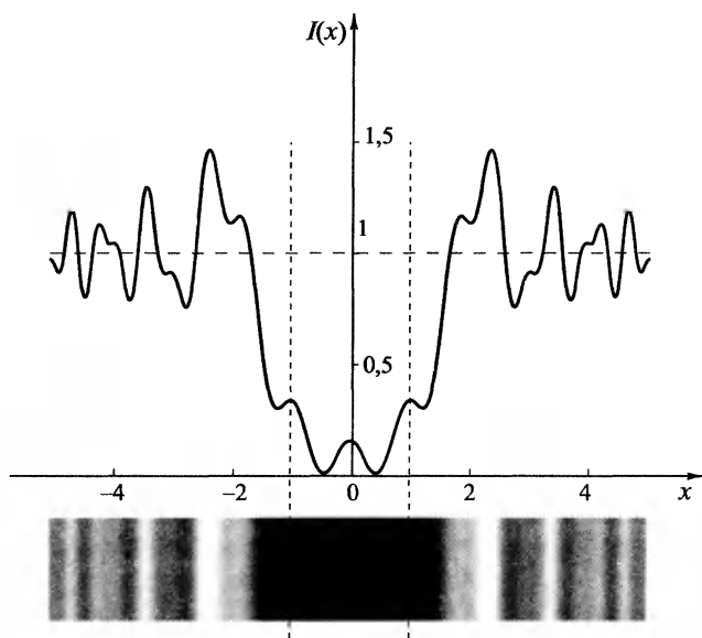
Рис. 6.14. Картина дифракции Френеля от тонкой проволоки
