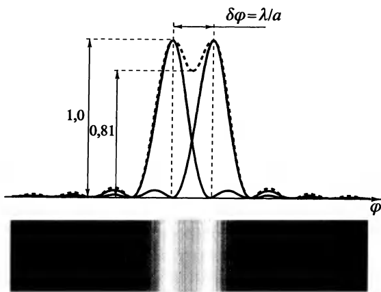
Рис. 6.39. Критерий Рэля
