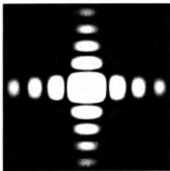
Рис. 6.22. Дифракция Фраунгофера от прямоугольного отверстия. Центральная область сильно переэкспонирована для выявления слабых побочных максимумов
