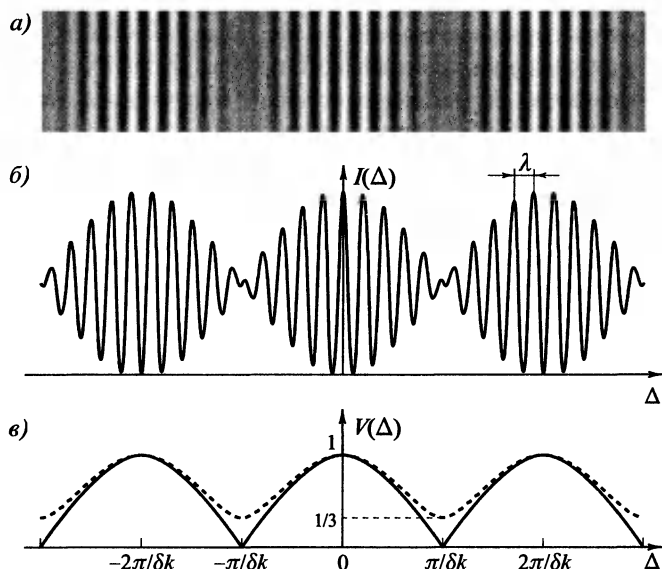
Рис. 5.15. Интерференционные полосы (а), график зависимости интенсивности от разности хода (б) и видность полос (в) двухлучевой интерференции в случае источника, излучающего две близкие спектральные линии. Штриховая линия соответствует источнику, у которого разность близких спектральных линий отличается вдвое
