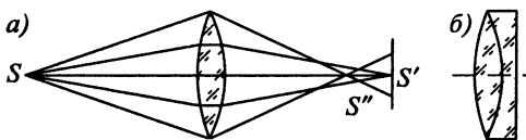
Рис. 7.22. Сферическая aberrация простой линзы (а) и сложная линза из разных сортов стекла, исправленная на сферическую aberrацию (б)
