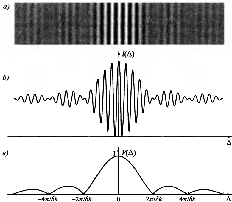
Рис. 5.16. Интерференционные полосы (а), график зависимости интенсивности от разности хода (б) и видность полос (в) двухлучевой интерференции в случае источника с прямоугольным спектральным контуром
