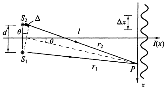
Рис. 5.4. К расчету интерференционной картины монохроматических волн, испускаемых двумя точечными источниками S_1 и S_2
