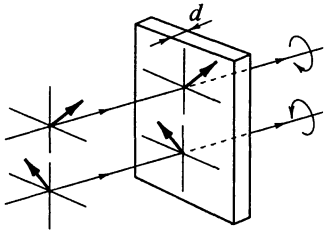
Рис. 4.4. Получение света круговой поляризации с помощью четвертьволновой пластинки
