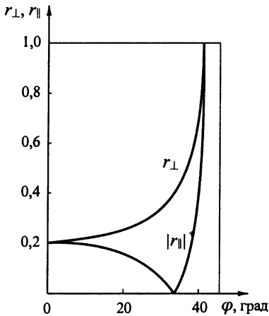
Рис. 3.8. Отношение амплитуд отраженной и падающей волн (в зависимости от угла падения) на границе стекло–воздух
