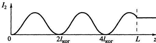
Рис. 10.2. Зависимость интенсивности второй гармоники от глубины проникновения в нелинейную среду
