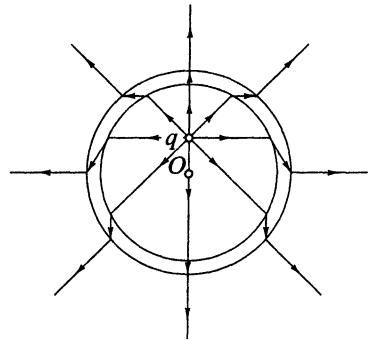
Рис. 1.14. Изломы силовых линий электрического поля заряда q , вызванные кратковременным ускоренным движением заряда вблизи точки O
