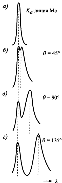
Рис. 9.15. Спектр рассеянного на графите излучения K_\alpha -линии молибдена
