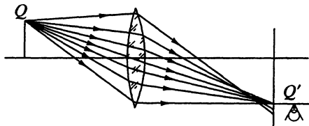
Рис. 7.23. К возникновению комы
