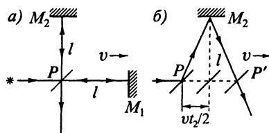
Рис. 8.3. Схема опыта Майкельсона
