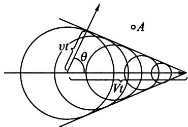
Рис. 2.18. Фронт ударной акустической волны в среде при движении снаряда со сверхзвуковой скоростью
