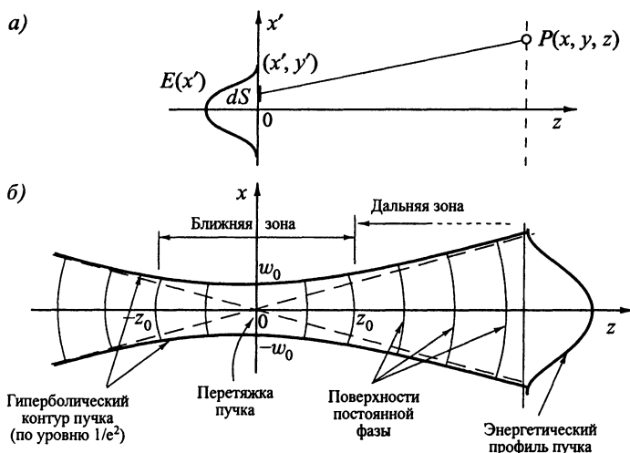
Рис. 6.27. Гауссов пучок: а — к расчету напряженности поля в точке P ; б — гиперболические границы пучка и волновые поверхности
