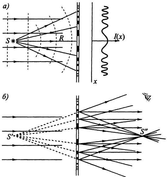
Рис. 7.36. Запись (а) и восстановление (б) голограммы точечного источника
