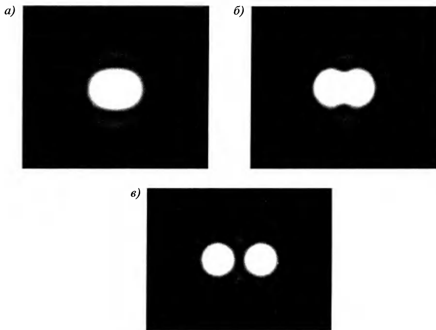
Рис. 7.32. Изображения двух близких точечных источников: а — согласно критерию Рэлея, источники не разрешены (расстояние между центрами дисков Эйри равно половине расстояния до первого минимума дифракционной картины); б — источники разрешены (расстояние между центрами равно расстоянию до первого минимума); в — расстояние между центрами равно расстоянию до второго минимума дифракционной картины.
