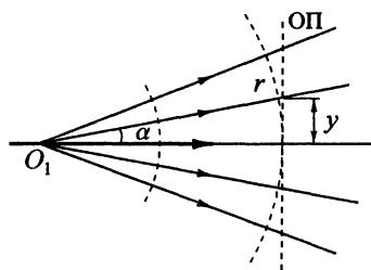
Рис. 7.14. Гомоцентрический пучок лучей
