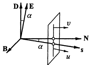
Рис. 4.6. Взаимное расположение векторов \mathbf{B} , \mathbf{D} , \mathbf{E} , \mathbf{N} и \mathbf{s} при распространении света в анизотропной среде
