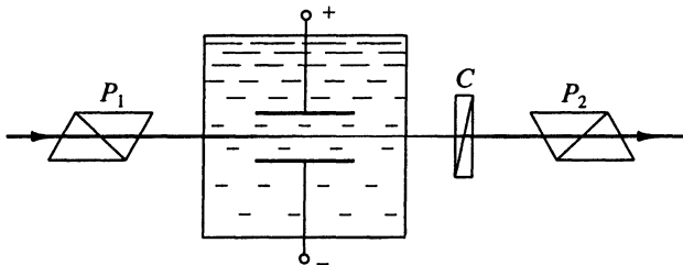
Рис. 4.15. Двойное лучепреломление в электрическом поле
