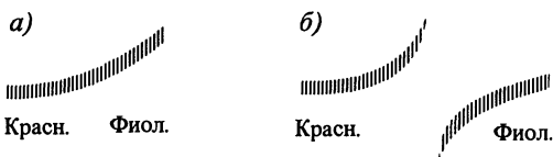
Рис. 2.3. Картина на экране, наблюдаемая в методе скрещенных призм. В случае нормальной дисперсии вещества призмы с горизонтальным ребром (стекло) показатель преломления растет с частотой и полоска монотонно поднимается от красного конца спектра к фиолетовому (а). Если вещество призмы обладает линией поглощения, полоска разрывается, а ее края изгибаются (б) в соответствии с ходом дисперсионной кривой на рис. 2.2
