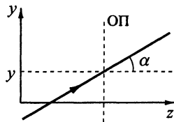
Рис. 7.6. Параметры y, \alpha меридионального луча
