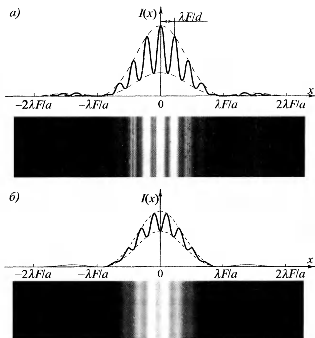
Рис. 6.26. Интерференционные полосы от двух щелей при освещении протяженным источником
