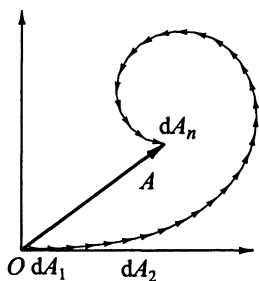
Рис. 6.10. Векторная диаграмма для результирующего колебания в точке наблюдения P от полосы волновой поверхности
