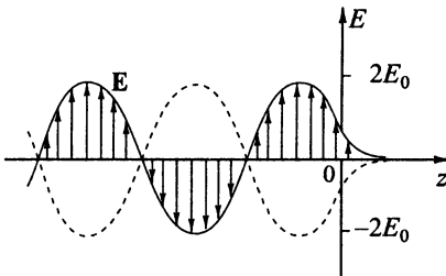
Рис. 3.15. Напряженность электрического поля световой волны при нормальном падении света на границу идеального металла
