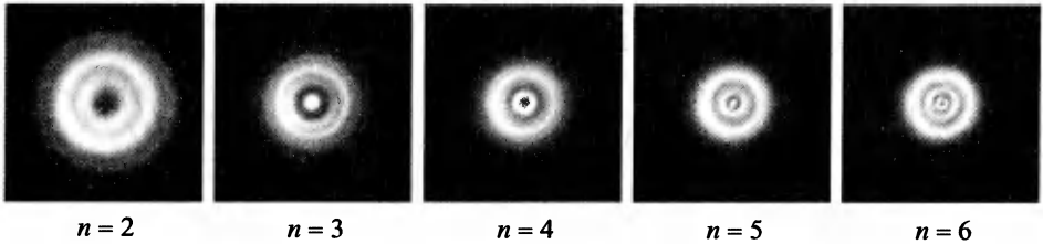
Рис. 6.5. Дифракционные картины от круглого отверстия, открывающего небольшое целое число зон Френеля. Фотографии выполнены С. К. Стафеевым
