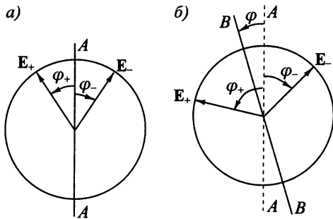
Рис. 2.8. Направление поляризации света: а — в точке z=0 ( AA ); б — в точке z=l ( BB )
