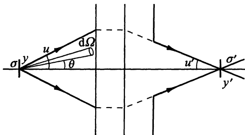
Рис. 7.28. К расчету освещенности изображения, формируемого оптической системой
