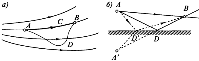
Рис. 7.3. К обоснованию принципа Ферма
