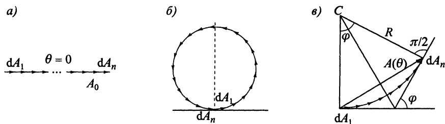
Рис. 6.19. Векторные диаграммы для дифракции Фраунгофера на щели
