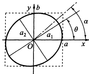
Рис. 1.8. Эллипс, описываемый концом вектора \mathbf{E} эллиптически поляризованной волны в фиксированной точке оси z
