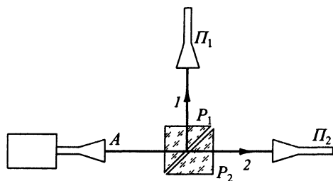
Рис. 3.10. Схема опыта, демонстрирующего нарушенное полное отражение в микроволновом диапазоне
