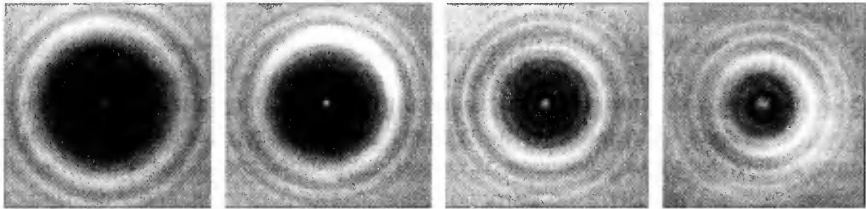
Рис. 6.6. Дифракционные картины от непрозрачного круглого диска. Число зон Френеля, перекрываемых диском, уменьшается слева направо. В центре геометрической тени диска наблюдается светлое пятно, называемое пятном Араго–Пуассона. Фотографии выполнены С. К. Стафеевым
