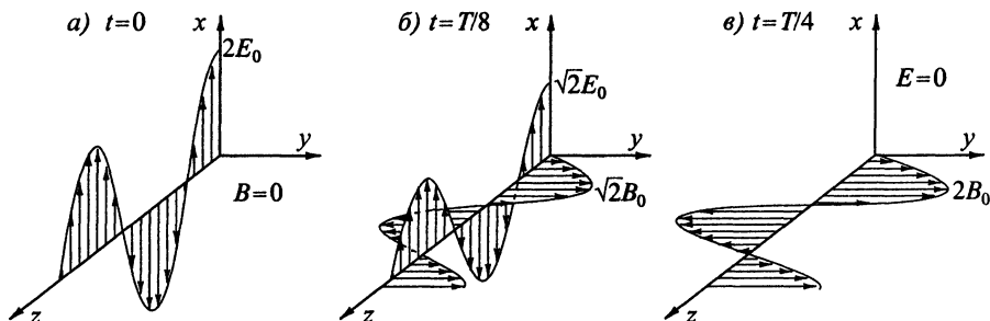
Рис. 1.11. Электрическое и магнитное поля стоячей линейно поляризованной волны в разных точках оси z для нескольких моментов времени
