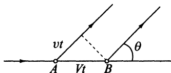
Рис. 2.19. К определению направления распространения излучения Вавилова—Черенкова
