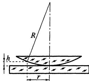
Рис. 5.13. К возникновению колец Ньютона
