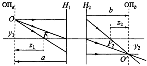
Рис. 7.13. Образование изображения в оптической системе
