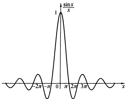
Рис. 1.22. График функции \frac{\sin x}{x}
