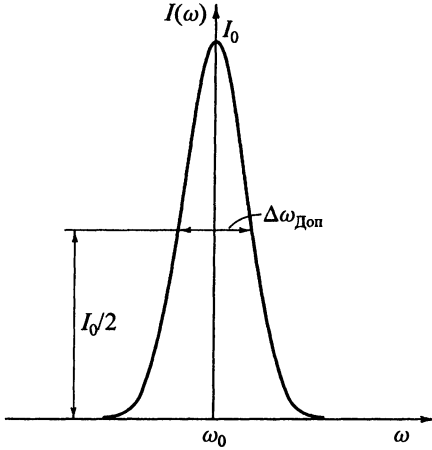
Рис. 1.24. Гауссов контур спектральной линии (неоднородное доплеровское уширение)
