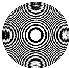
Рис. 6.7. Зонная пластинка Френеля
