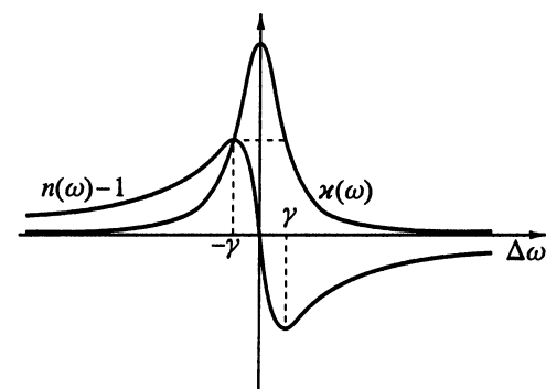
Рис. 2.2. Дисперсионная кривая и лоренцевский спектральный контур линии поглощения. В пределах ширины контура 2\gamma показатель преломления n(\omega) - 1 уменьшается с увеличением частоты (аномальная дисперсия)
