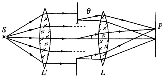
Рис. 6.16. Схема наблюдения дифракции Фраунгофера в фокальной плоскости собирающей линзы
