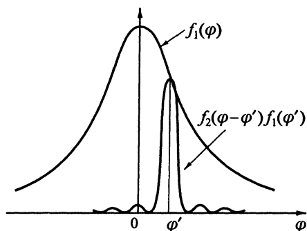
Рис. 6.38. К нахождению результирующего аппаратного контура
